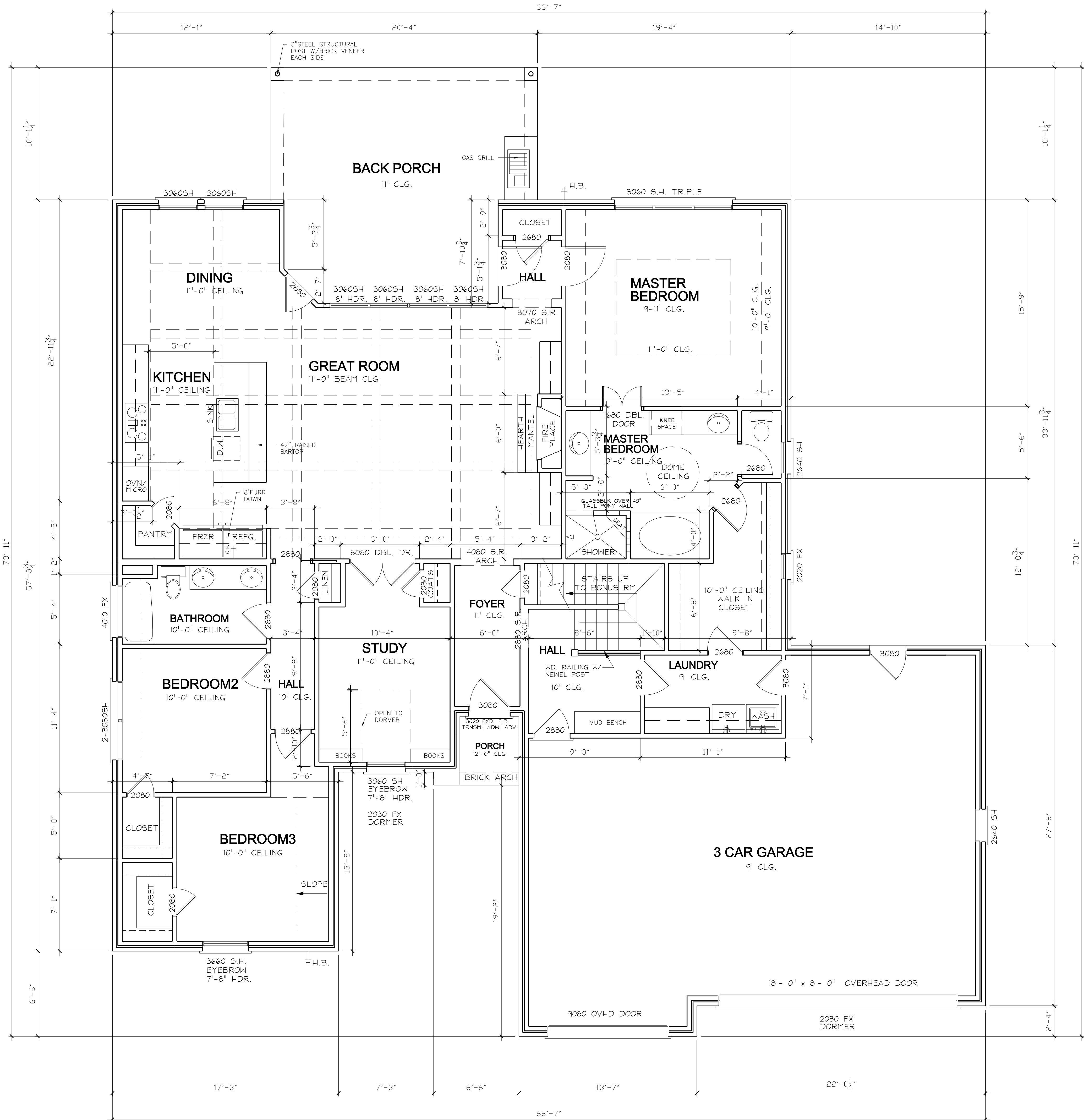
FLOORPLAN 1/4"=1'-0"
